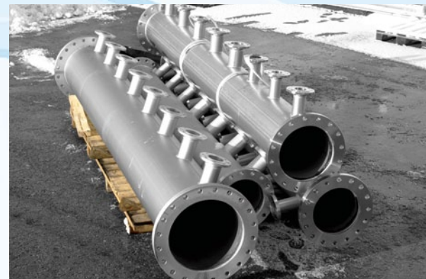
Projekt Dubai: Verteiler DN500, DN300, DN150 für Trinkwasser
