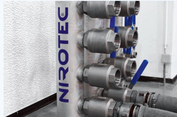
Projekt Waidhofen: Standrohr DN150 mit 3" Kugelhähnen
