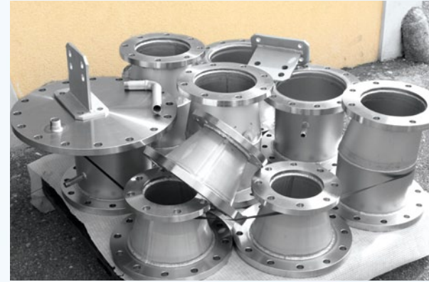
FF-Stücke und FFR-Stücke, DN80 und DN100
