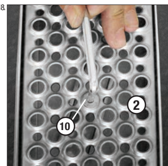
Roste mit Rinne-Module fixieren
