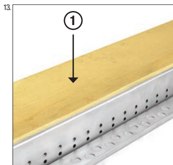
Holzstaffel einlegen (Bauzeitenschutz)
