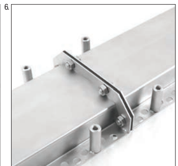
Endstück mit Rinnenmodul verschrauben
