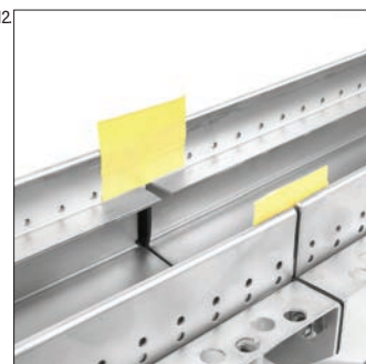
Flanschspalten und Endstücke abkleben
