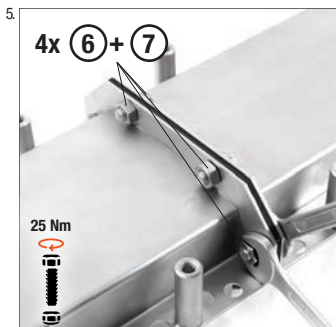
Rinnenmodule verschrauben
