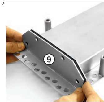
Endstück positionieren
