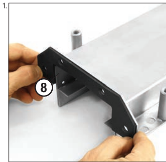
Dichtung für Endstück anlegen
