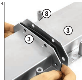
Flanschdichtung zwischen Rinnenmodule einlegen
